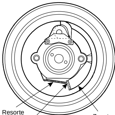
Resorte Agujero No. 2 Zapata de freno (Dibujo MHP1369E)
